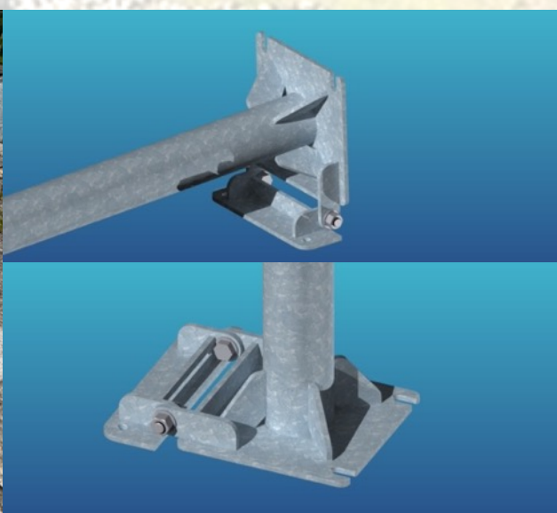
Poteau sur platine articulée (zone inondable)
