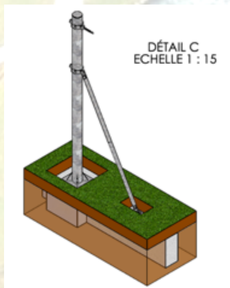
Poteau en acier galvanisé dimensions sur mesures Avec ou sans jambe de force
